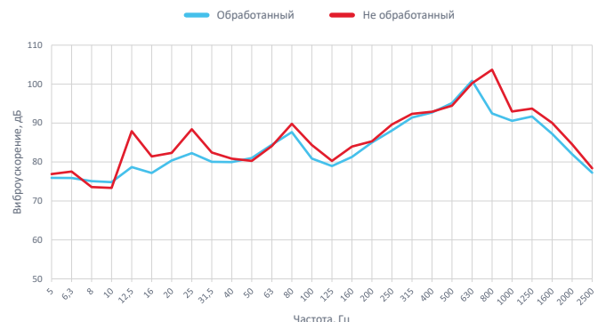
Уровни вибрации на полу в автомобиле Ford Focus при проезде грузового фургона в попутном направлении со скоростью 100км/ч
