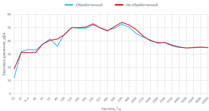
Уровни шума на месте водителя в автомобиле Ford Focus при проезде грузового фургона в попутном направлении со скоростью 80км/ч
