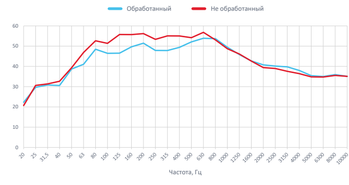
Уровни шума на месте заднего ряда сидений в автомобиле Ford Focus при проезде грузового фургона в попутном направлении со скоростью 100км/ч
