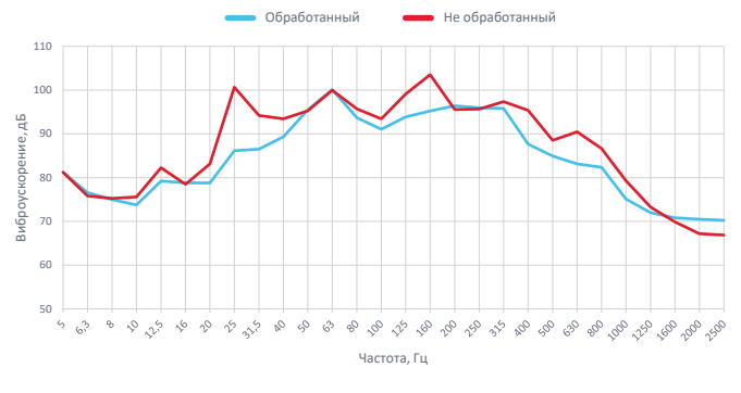
Уровни вибрации на обшивке левой задней двери в автомобиле Ford Focus при проезде грузового фургона в попутном направлении со скоростью 80км/ч
