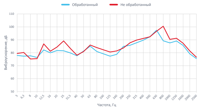
Уровни вибрации на полу в автомобиле Ford Focus при проезде грузового фургона в попутном направлении со скоростью 80км/ч
