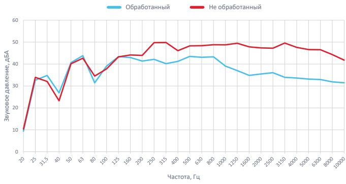
Уровни шума между передними сиденьями в автомобиле Ford Focus при проезде грузового фургона во встречном направлении
