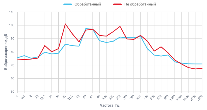
Уровни вибрации на обшивке левой задней двери в автомобиле Ford Focus при проезде грузового фургона во встречном направлении
