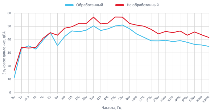
Уровни шума между передними сиденьями в автомобиле Ford Focus при проезде грузового фургона в попутном направлении со скоростью 80км/ч
